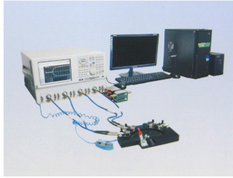
TDR & NA tester
